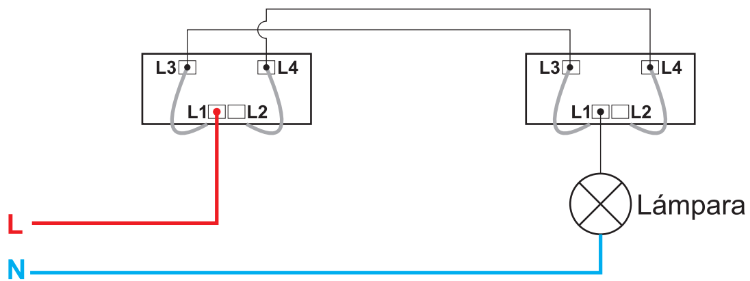
ESQUEMA DE CONEXIÓN MODO COMBINACIÓN
